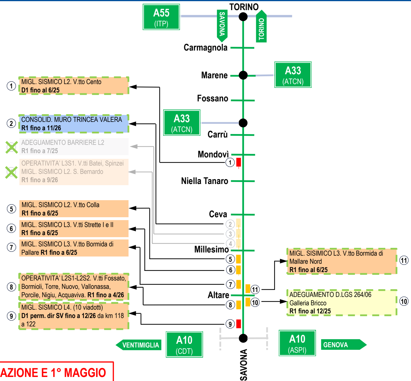
Configurazione FERIAI o festivi nella dir. di traffico minore
