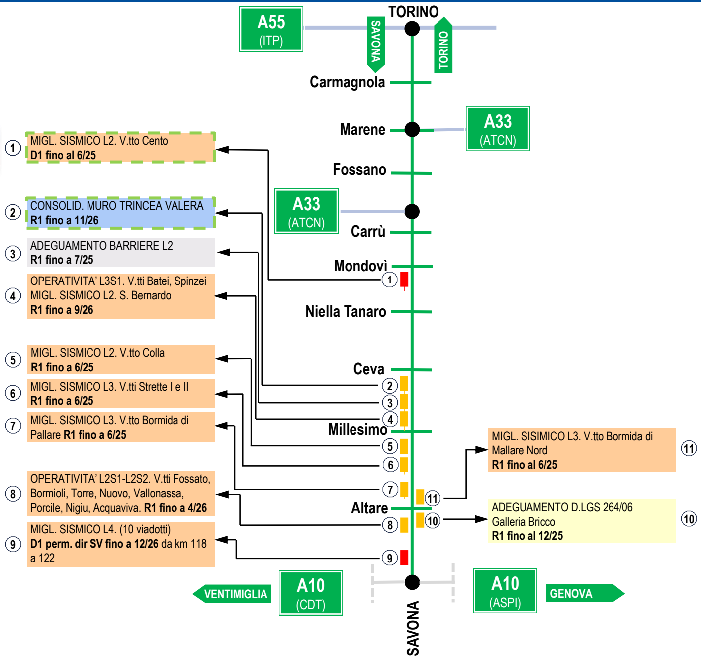
Configurazione FERIAI o festivi nella dir. di traffico minore
