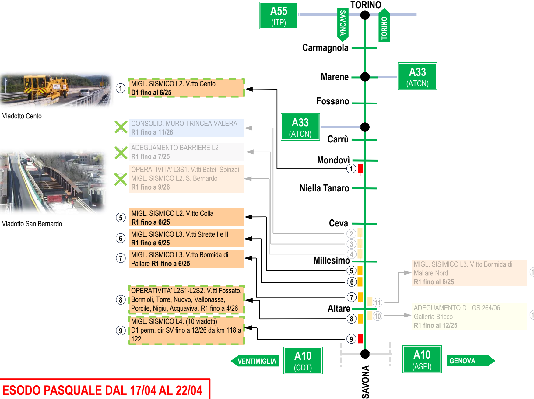
Configurazione FERIAI o festivi nella dir. di traffico minore
